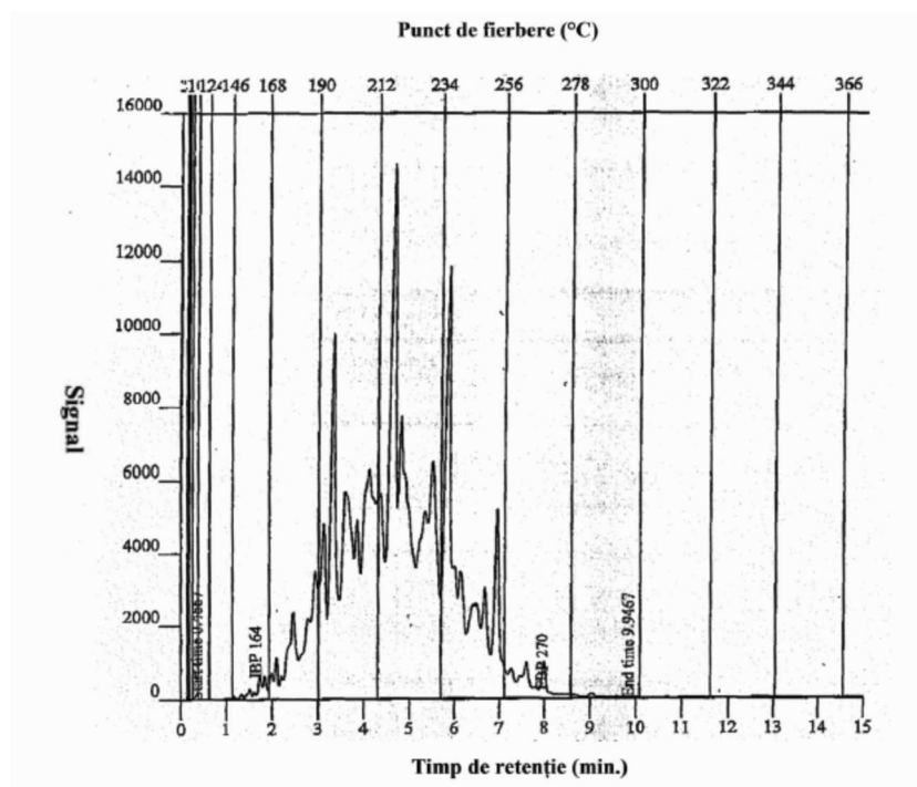
Corelare EN ISO 3405 (echivalentă cu metoda ASTM D 86) (STP 577) - distribuție
